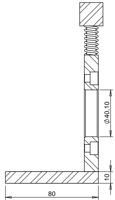
COUPE A-A
